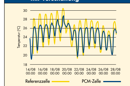
Abb 7: Wandtemperaturverlauf in den Leichtbauzellen über zwei Wochen mit Verschattung
