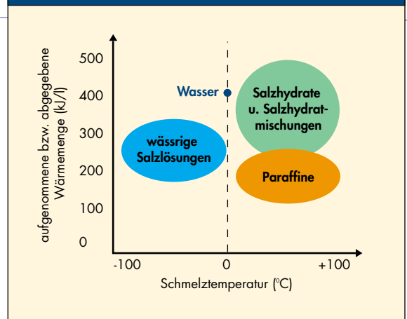
Abb 3: Typische Phasenübergangstemperaturen verschiedener PCM-Substanzklassen
